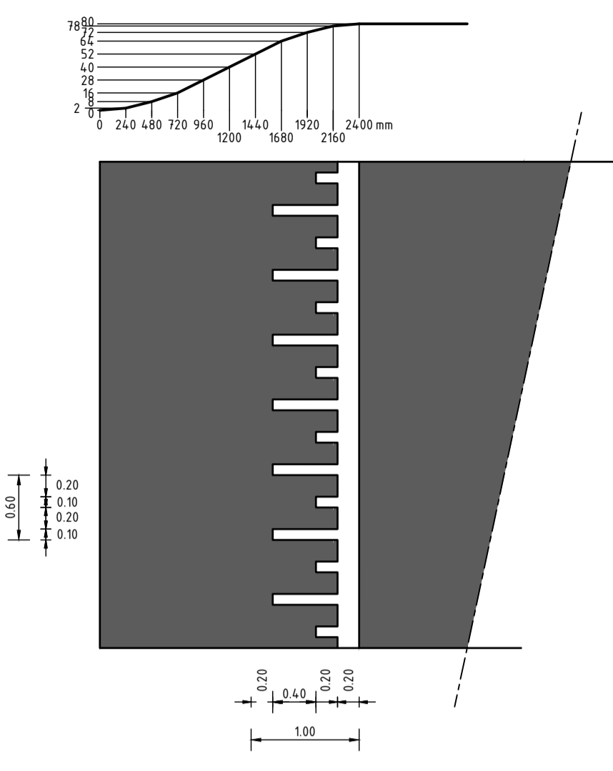
Detail, plateauoprit, 50km/u met marking 30km/u Schaal 1:50
