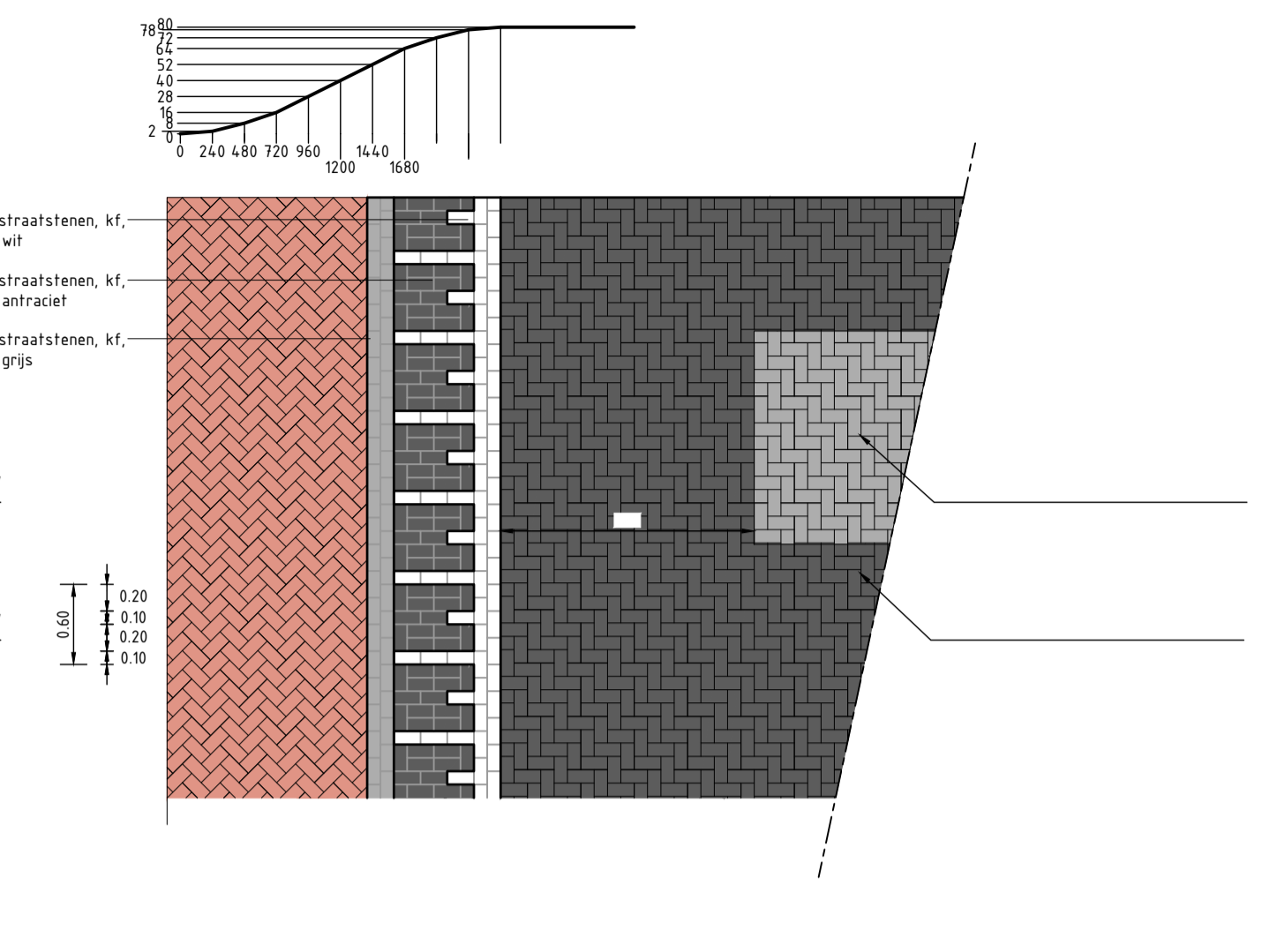
Detail, plateauoprit, 50km/u - met marking 30km/u Schaal 1:50
