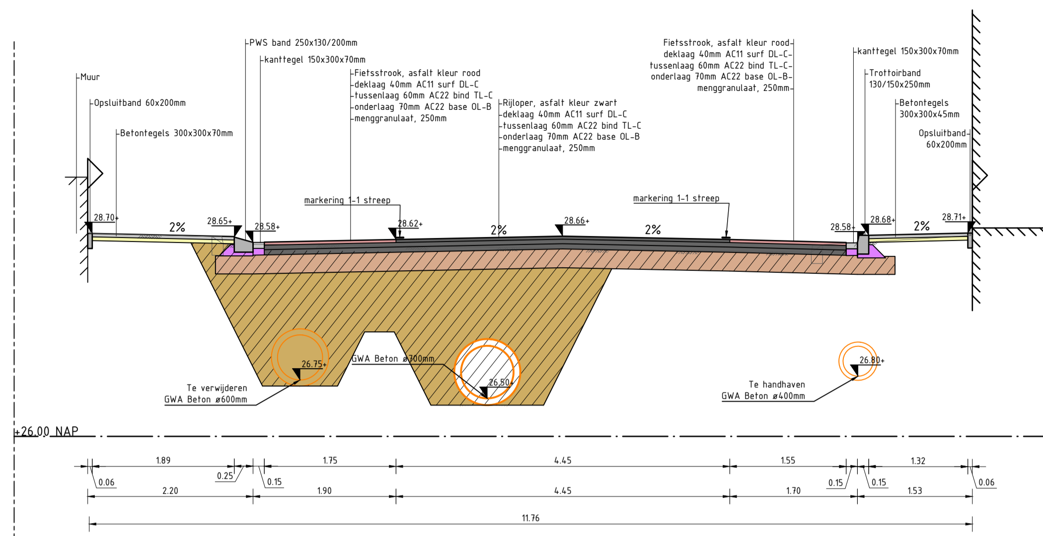
Profiel A-A Schaal 1:50
