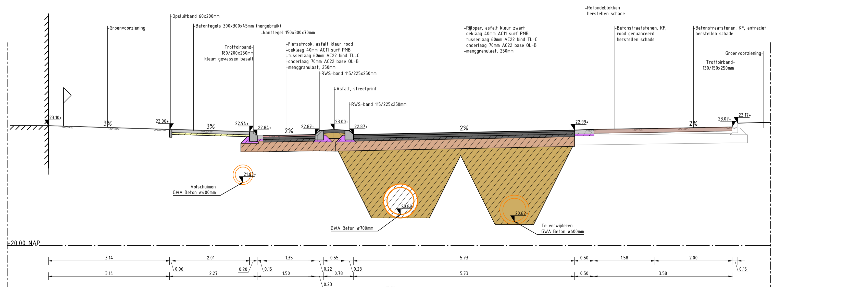
Profiel B-B Schaal 1:50
