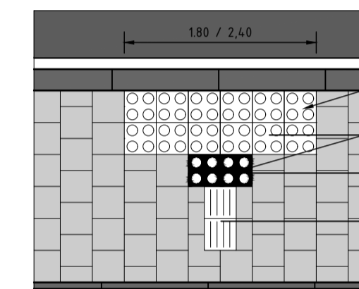
Principedetail 3: oversteek gidsgeleidetegels Schaal 1:50
